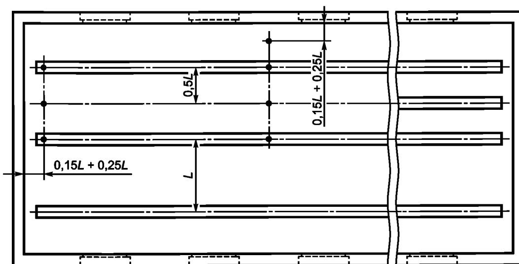
Рисунок Б.1 — Расположение контрольных точек при измерении минимальной освещенности помещения от светильников, принимаемых за точечные излучатели
